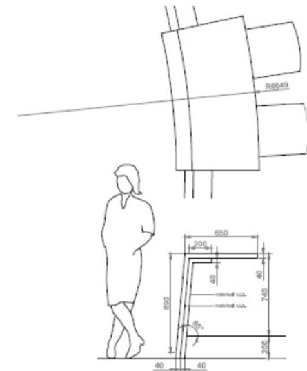
Zijaanzicht bureau regie
