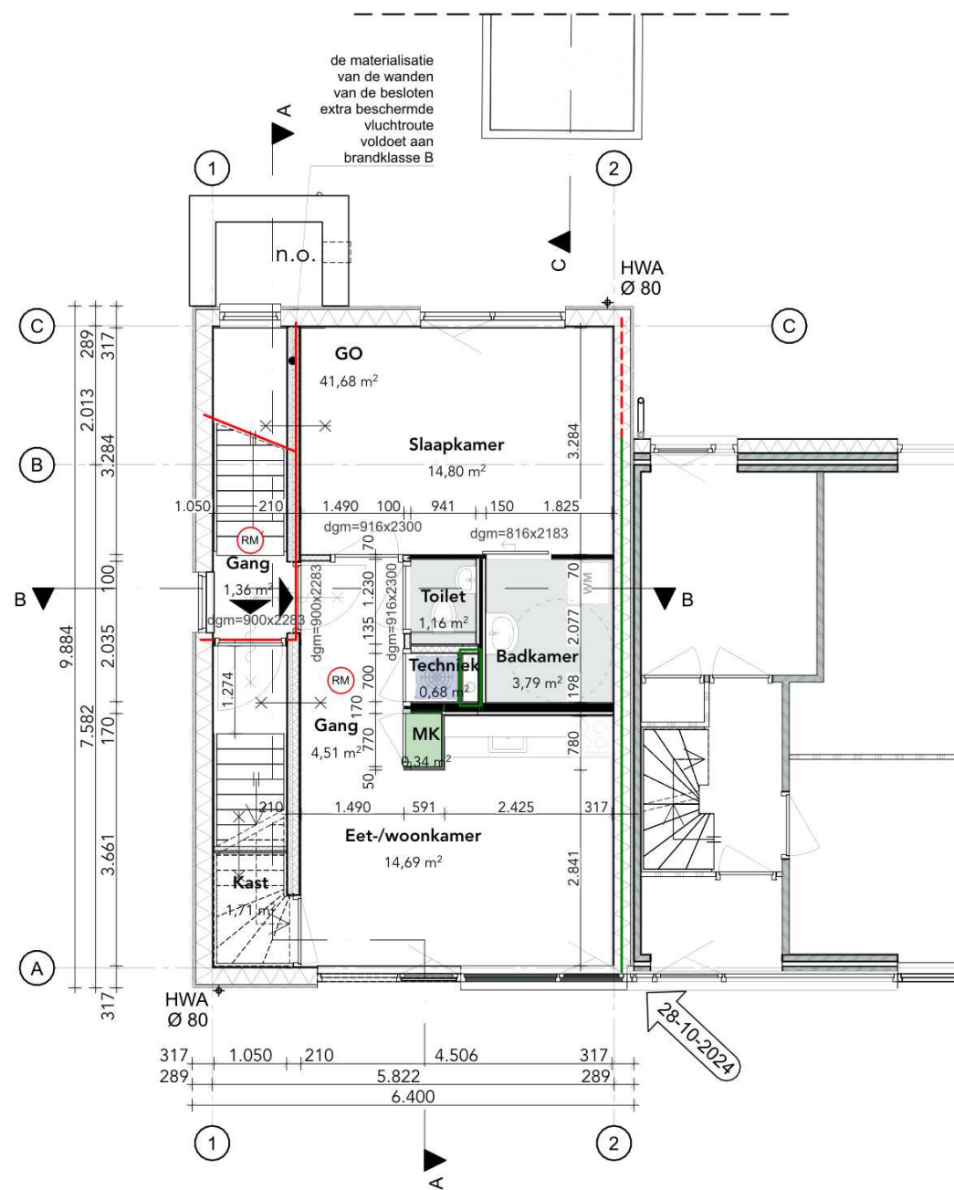
eerste verdieping
