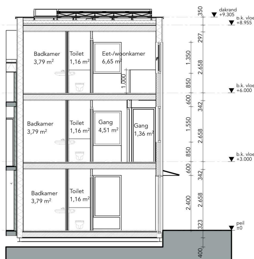
Doorsnede B
