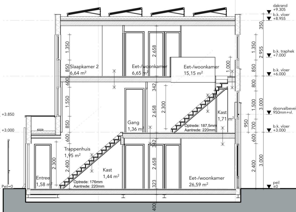
Doorsnede A
