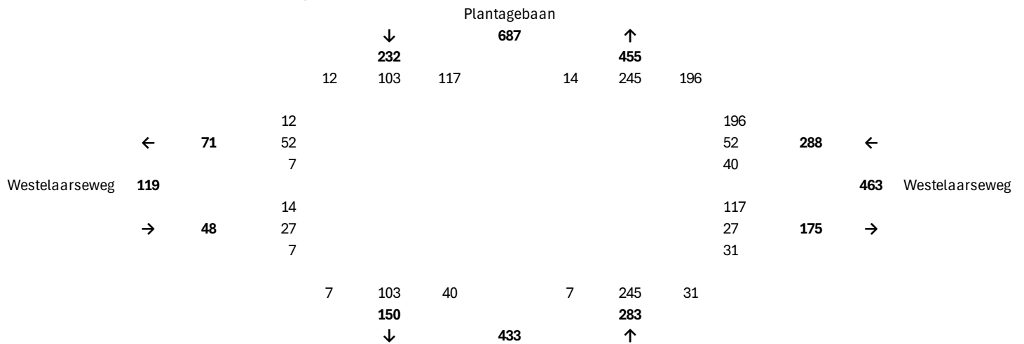
Figuur 5: gemiddelde drukste ochtendspitsuur intensiteiten per rijrichting
